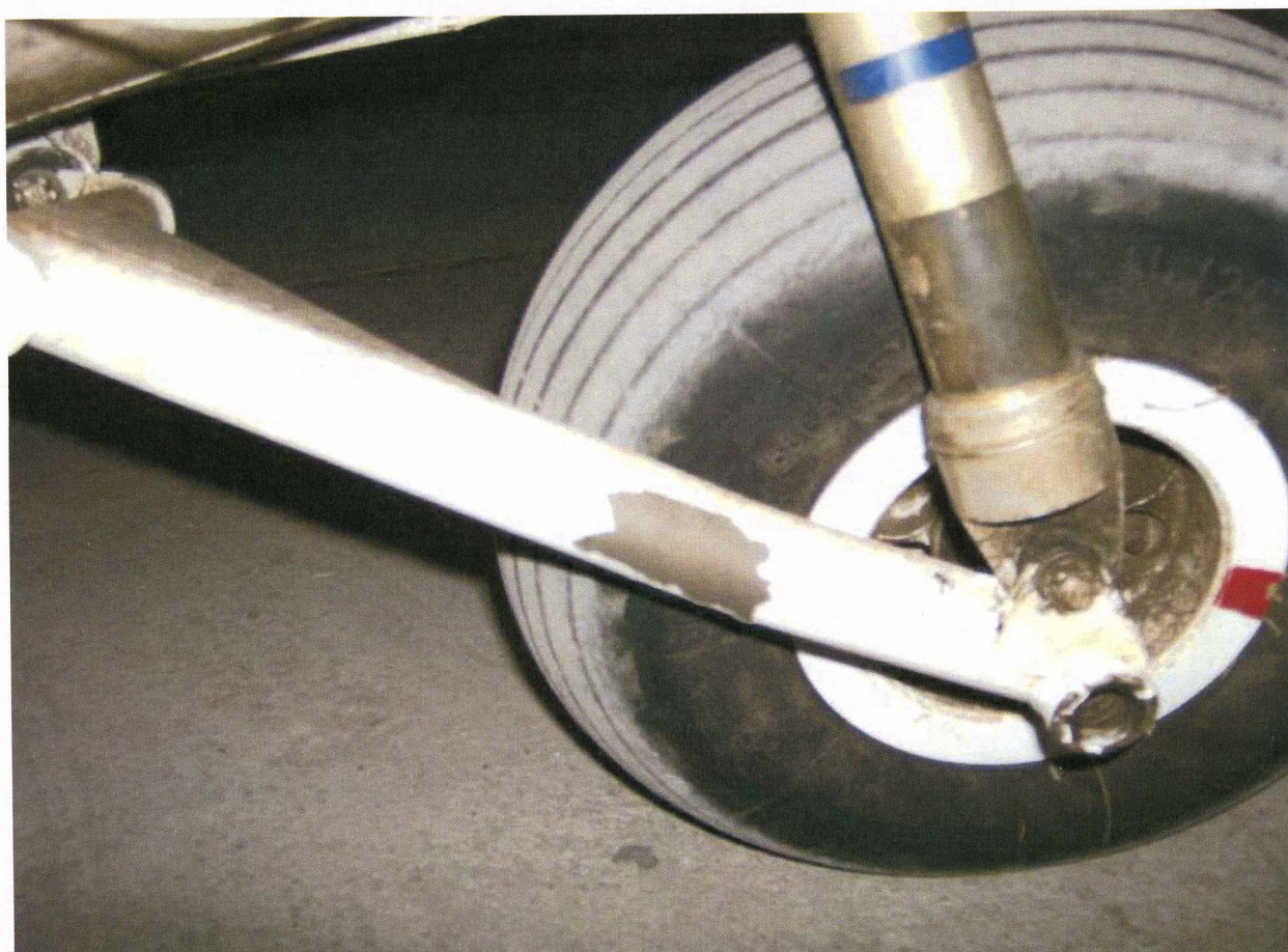
3 i 4 – Uszkodzone podwozie, lewa strona – zbliżenie. Zdjęcie dolne z oznakowaniami uszkodzeń.
