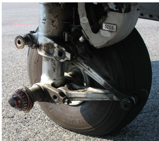
Fot.6a i 6b – Widoki uszkodzonego podwozia przedniego.
