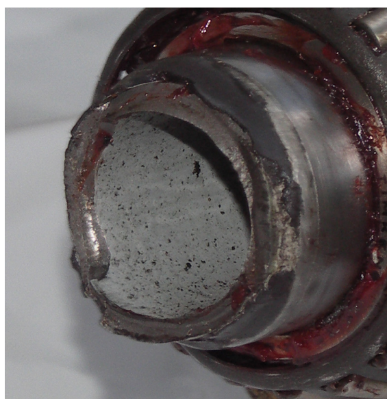
Fot.10a i 10b – Przełom zakończenia osi w różnym oświetleniu, widoczne resztki gumowej opaski ochronnej.
